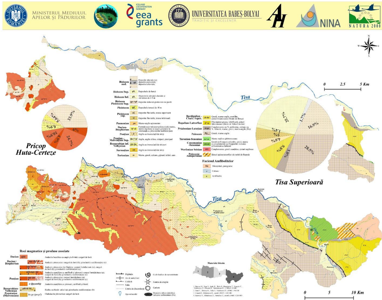
Figura 1 . Harta geologică a siturilor Natura 2000 Pricop-Huta Certeze și Tisa Superioară
